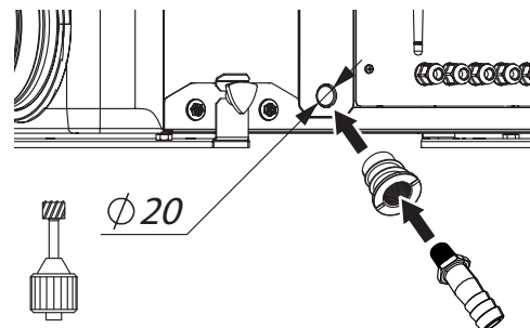
Instalacja przyłącza odpływowego przy montażu urządzenia zgodnie ze schematami 2-4
