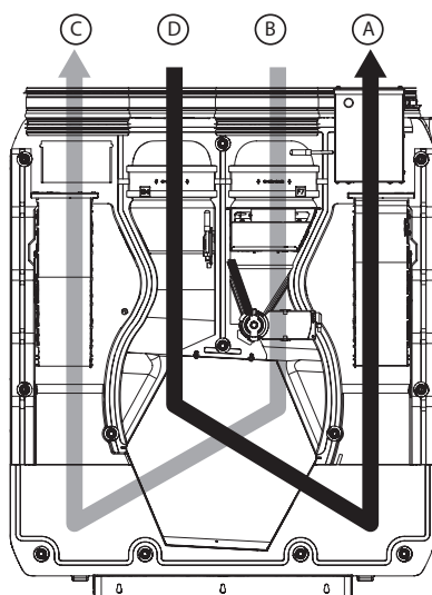
Reneo S(E) 350/550(-E) VG A – wyrzutnia, B – czerpnia, C – nawiew, D – wywiew
