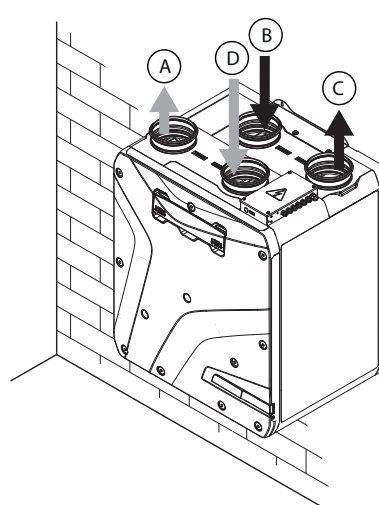
Reneo S(E) 350/550(-E) VG - po zamianie strony serwisowej
