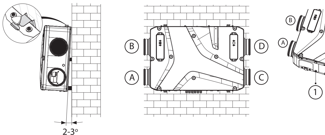
A – wyrzutnia, B – czerpnia, C – nawiew, D – wywiew, 1 – otwór odpływowy Schemat 4. Montaż ścienny, poziomy
