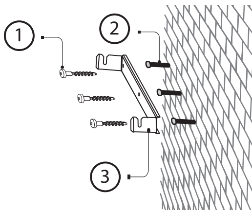
1 – śruba, 2 – kołek rozporowy, 3 – wspornik montażowy;
